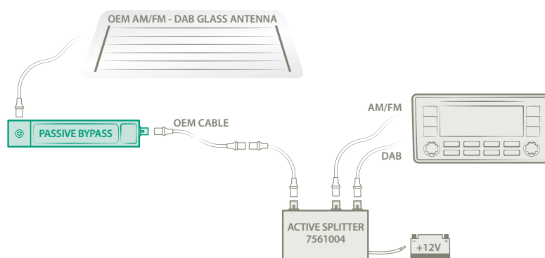
Mounting scheme / Schema di montaggio
